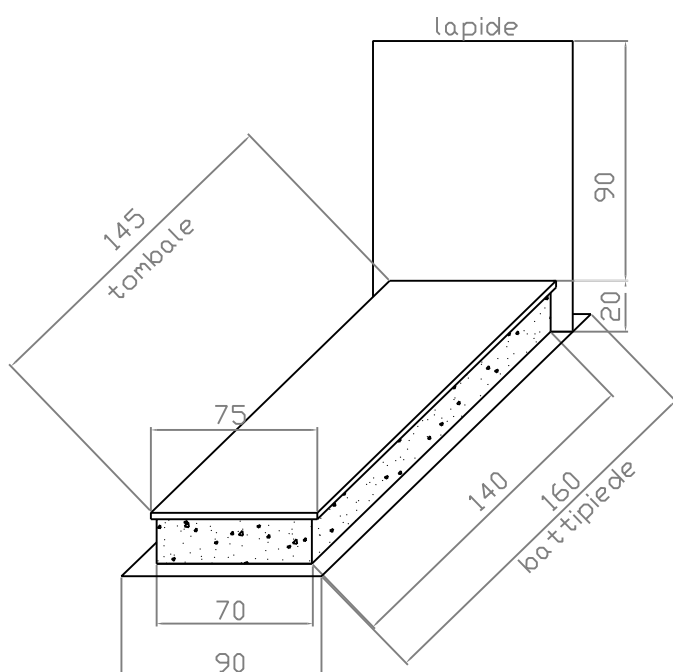
VISTA ASSONOMETRICA
