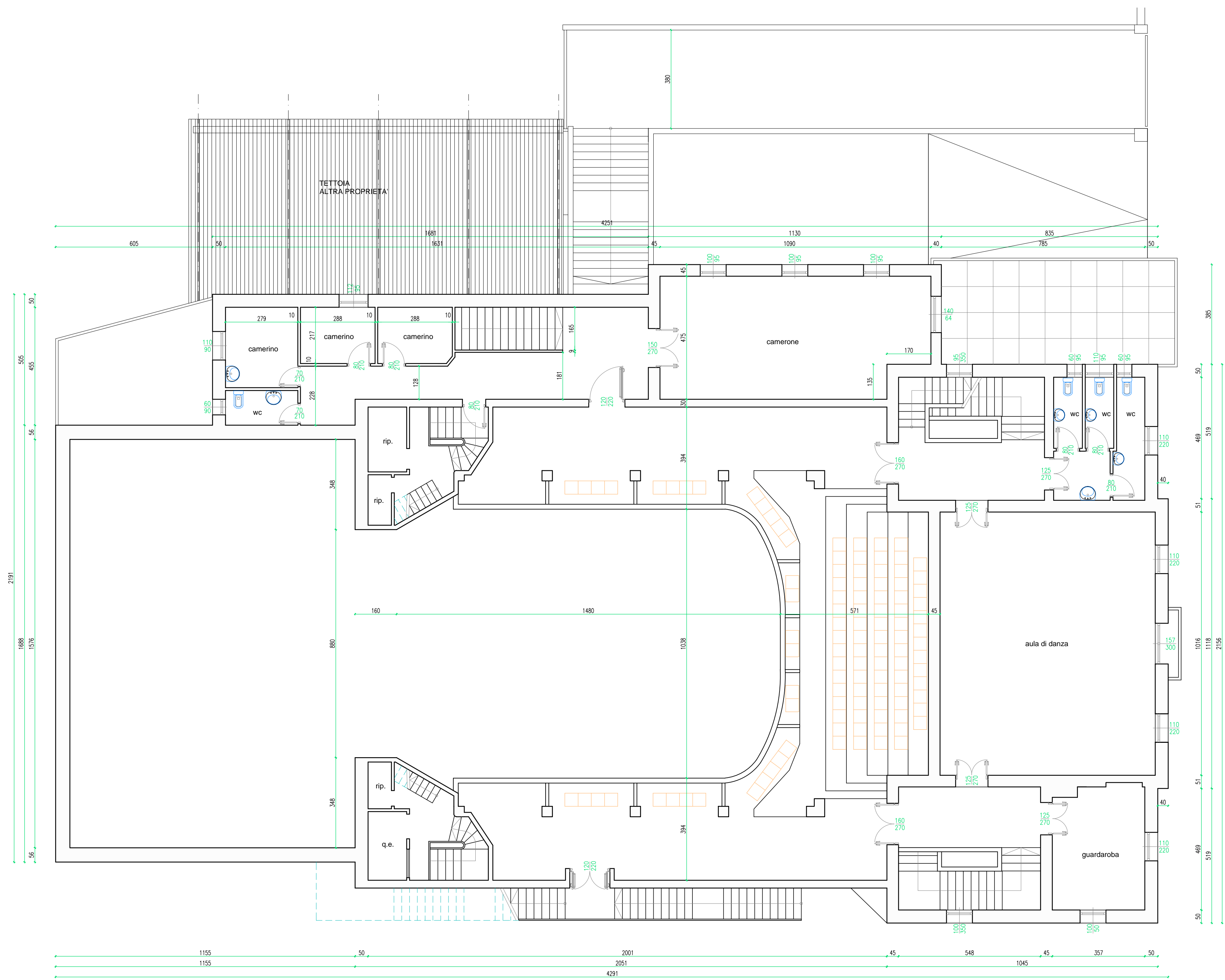
Piano primo
