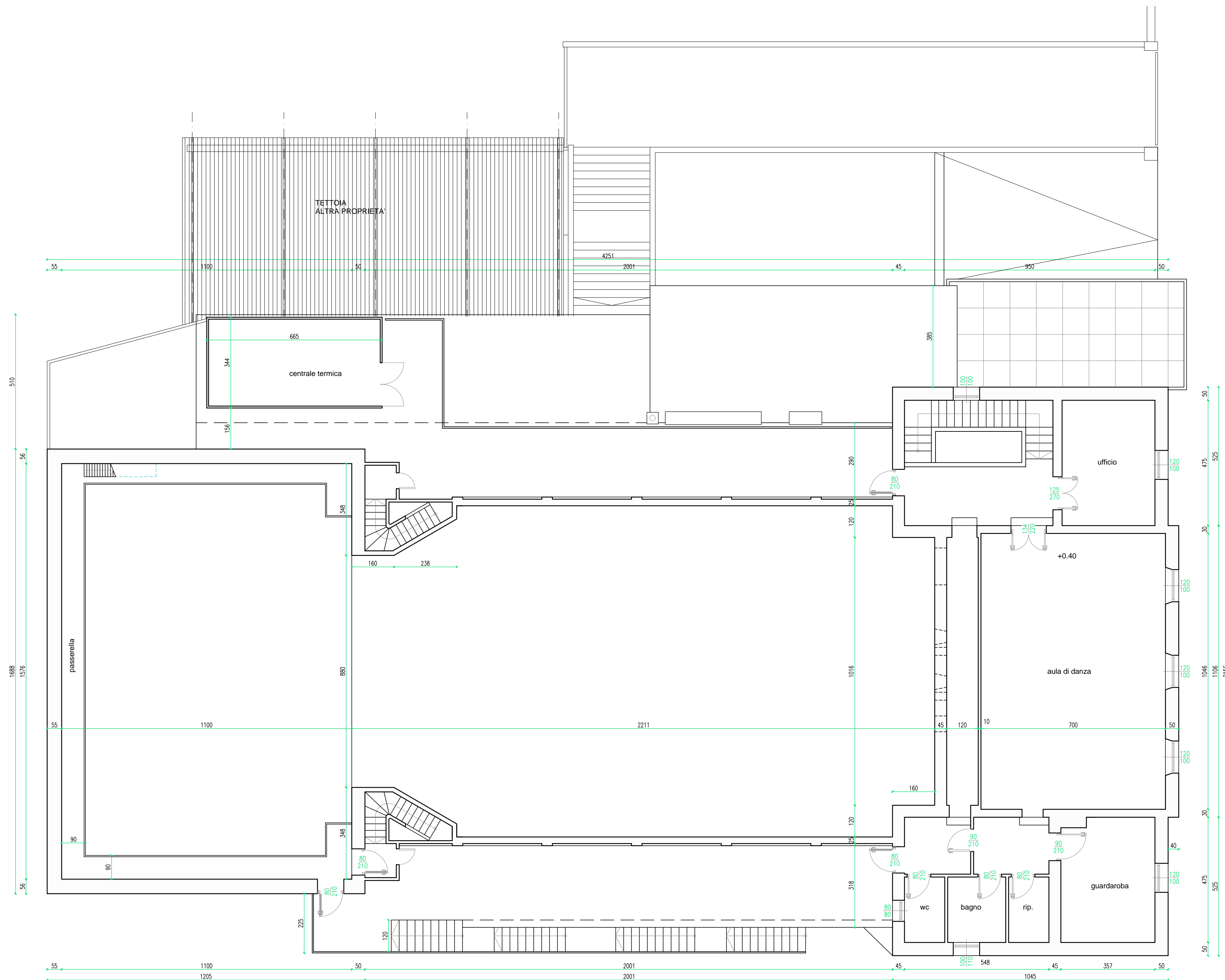
Piano secondo
